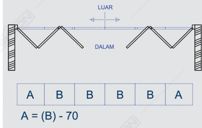
Gambar Tampak Atas
