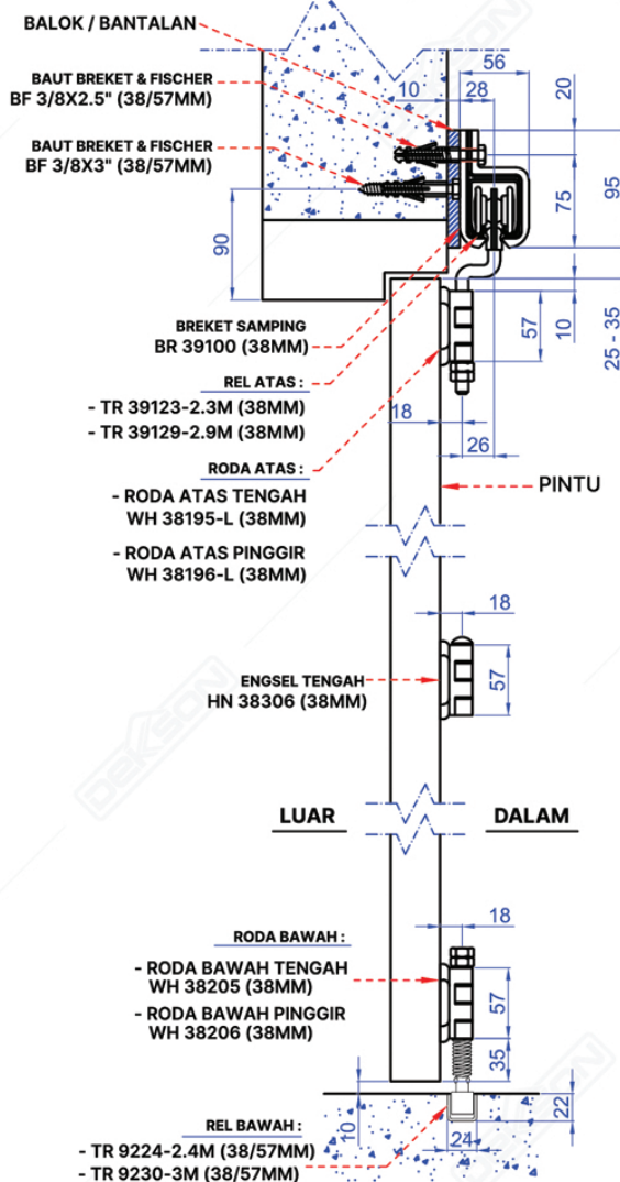
Gambar Potongan
