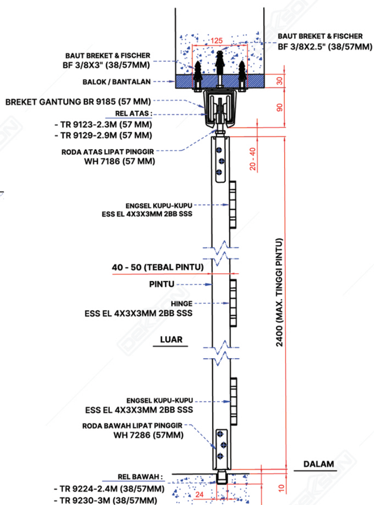
Gambar Potongan
