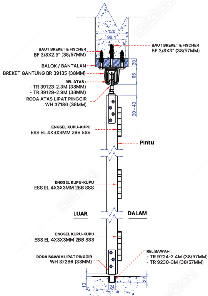
Gambar Potongan
