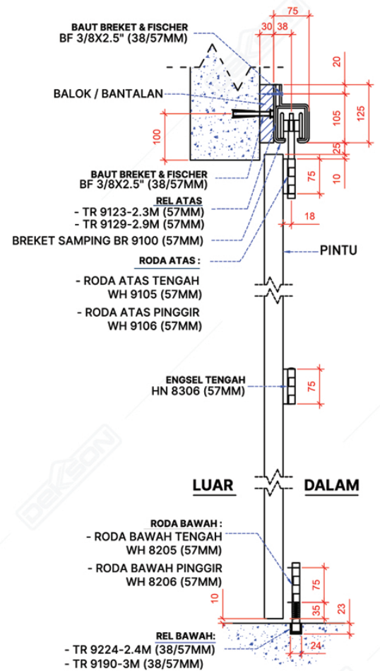
Gambar Potongan
