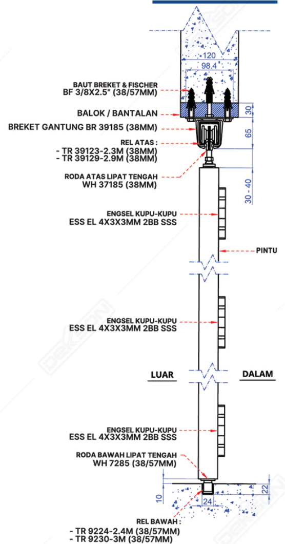
Gambar Potongan
