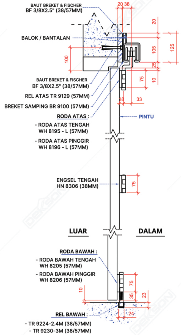
Gambar Potongan
