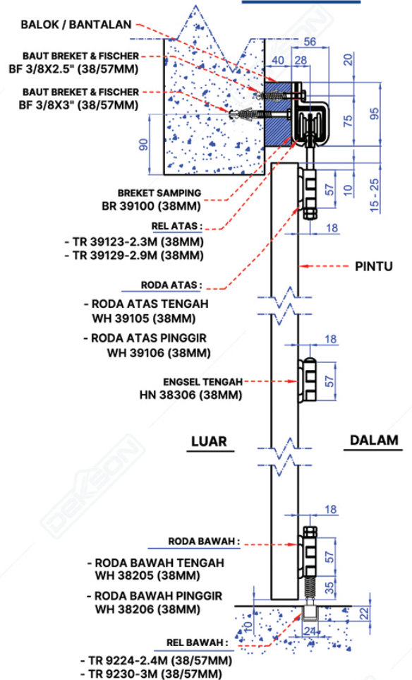
Gambar Potongan
