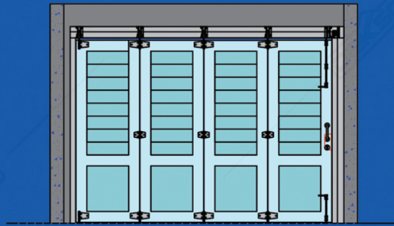
GAMBAR TAMPAK DEPAN
